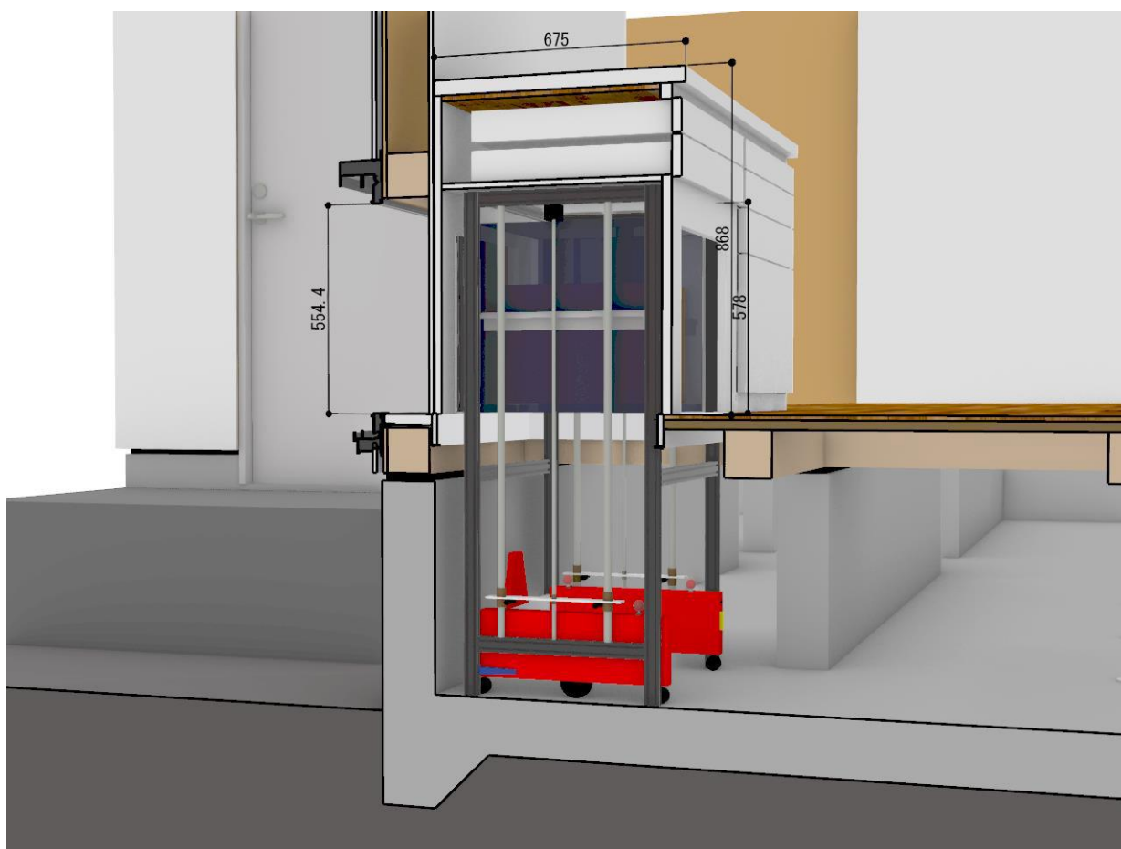
▼システム組み込み (D650mm)
