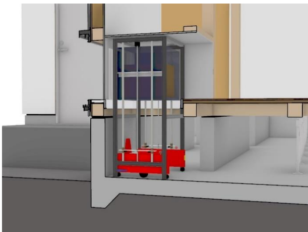
▼柱間外周寄せ (柱芯 910mm)
