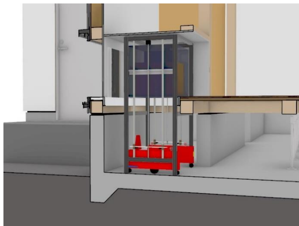
▼柱間内寄せ (柱芯 910mm)
